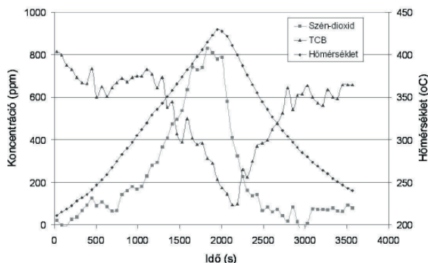
2. Ábra. Triklór-benzol katalitikus bontása közben a TCB és CO 2 koncentrációjának változása a vizsgálat idejének és a hőmérséklet függvényében
