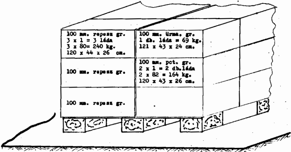
5.sz. ábra Rakodólapra pántolt ládázott lösszer
