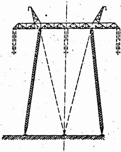
1. ábr. 750 kV-os kikötési tartószerlep
