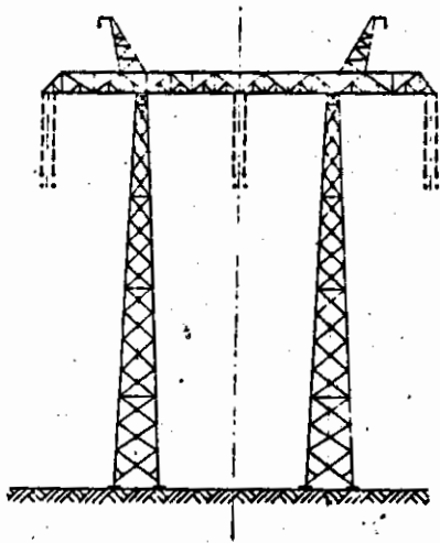
2. ábr. 750 kV-os átkerülő tartószerlep
