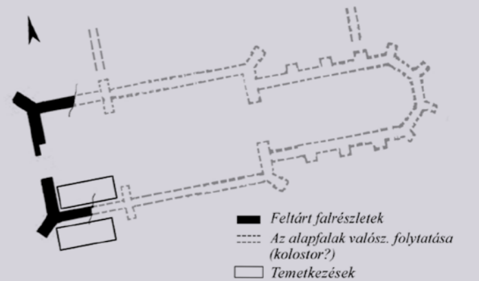
▲ A klastrompusztai (fent, helyszíni táblán) és a pilisszántói templom alaprajzai (alább, Z.T.Cs.)
