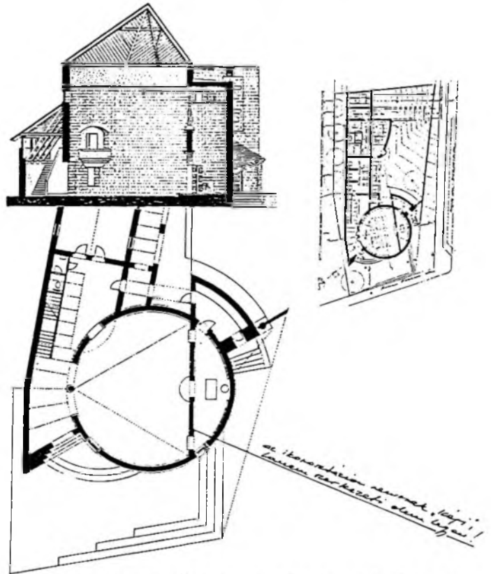
Kazincbarcika, görög katolikus templom, alternatív terv
