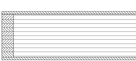
2. ábra – 9 fóliás panel, légrések vastagsága 3 mm
