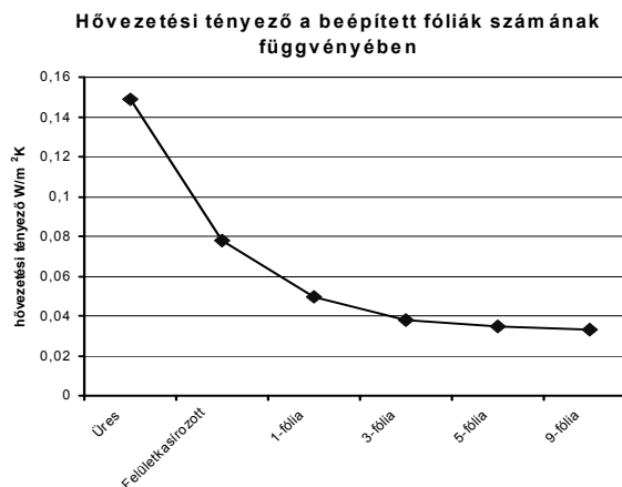
3. ábra – Tükörpanel kísérletsorozat eredményei
