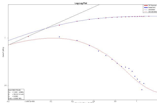
2. ábra: Log – Log (diagnosztikai) ábra
