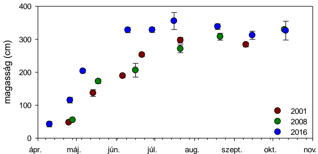
2. ábra. A nád ( Phragmites australis ) növekedése a Balatonban 2001, 2008, 2016-ban.
