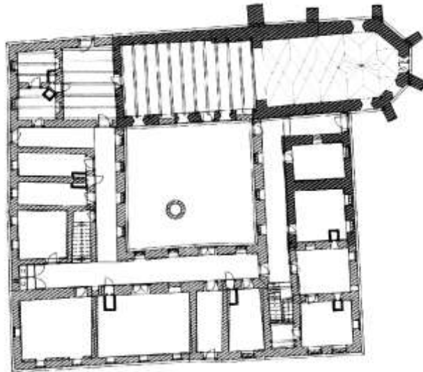
A (szent)jakab-hegyi kolostor alaprajza (Buzás Gergely nyomán F. Romhányi 2010)
