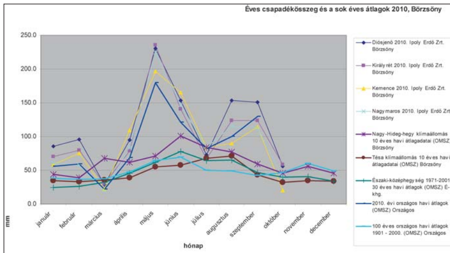
Éves csapadékösszeg mérőállomásonként, 2010 októberig, szerk.: Nagy L., Ipoly Erdő Zrt.
