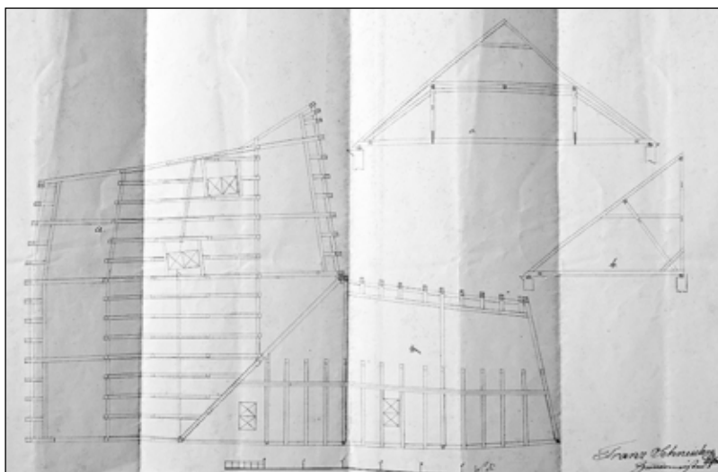
5. kép. Új fedélszék terve. Schneider Ferenc [1841?] (MNL OL)
