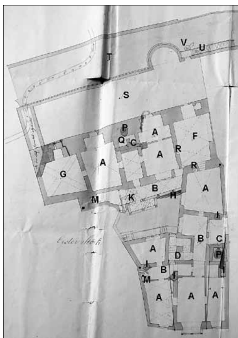
2. kép. Az első emelet alaprajza (részlet). Handler József, 1822 (MNL OL)
