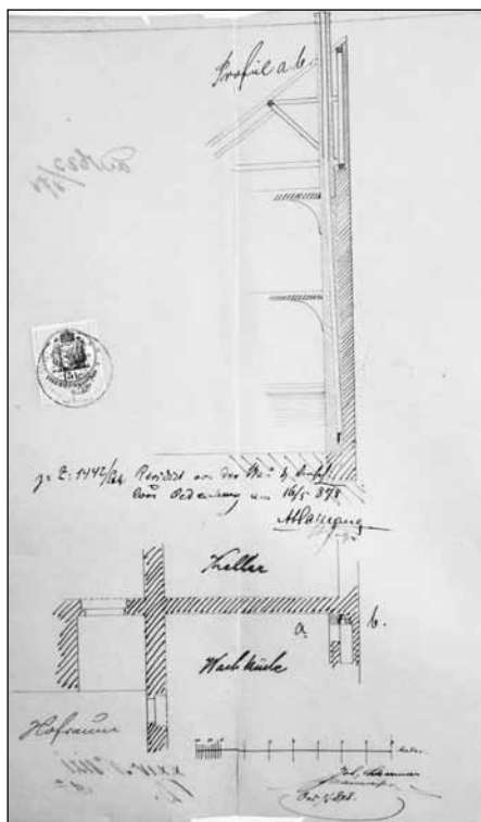
7. kép. Kémény terve. Schármár János, 1878 (MNL GyMSMSL)
